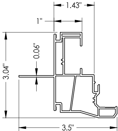
3 FRAME JAMB
